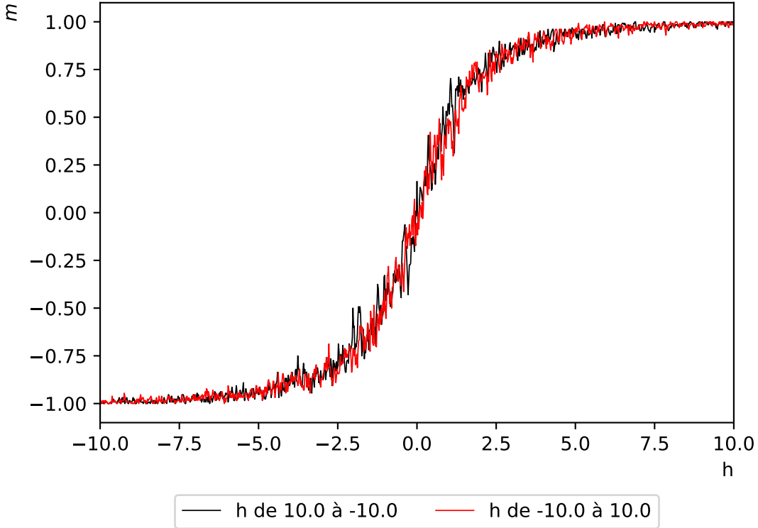
Hystérésis de l'aimantation - réseau de taille L=16 - champ magnétique d'amplitude h=10 à T=5.0
